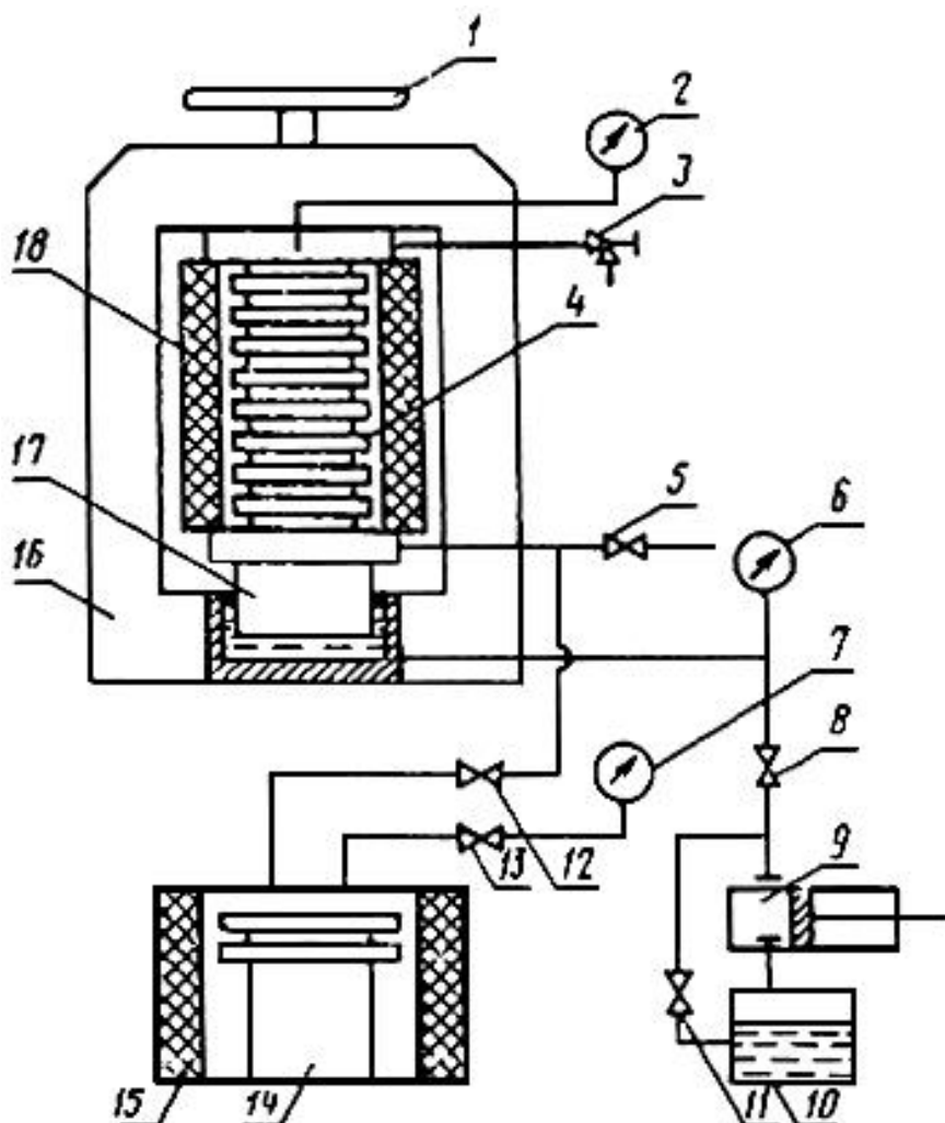
Схема автоклава типа АП-1
